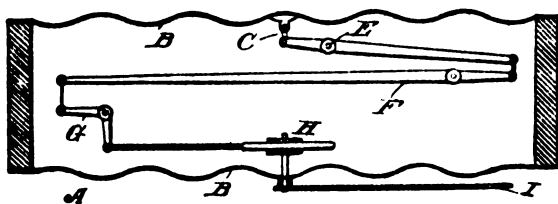
Fig. 74. Aneroid Barometer
